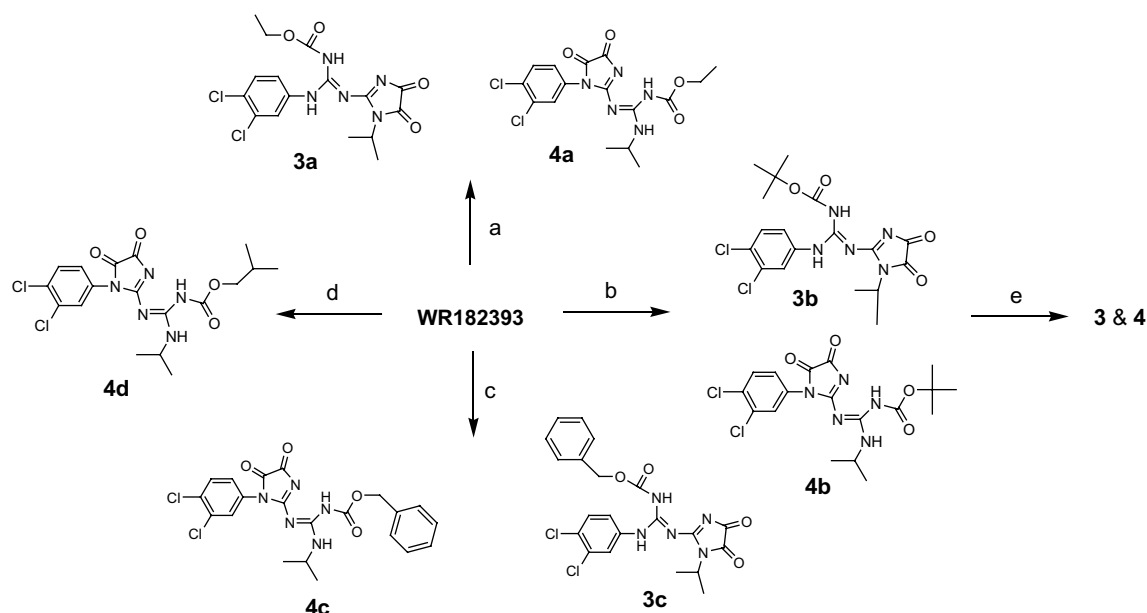
Scheme 2. Reagents: (a) \text{ClOCOEt} , \text{Et}_3\text{N} , \text{CHCl}_3 ; (b) di- t -butyl-dicarbonate, DMAP, \text{CHCl}_3 ; (c) dibenzylidene dicarbonate, DMAP, DMF; (d) \text{ClOCOCH}_2\text{CH}(\text{CH}_3)_2 , \text{Et}_3\text{N} , \text{CHCl}_3 ; (e) 3 N HCl/EtOAc.
